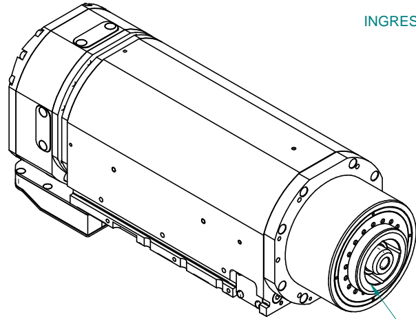
ATTACCO HSK 63E DIN 69893-5 TOOL INTERFACE HSK 63E DIN 69893-5
